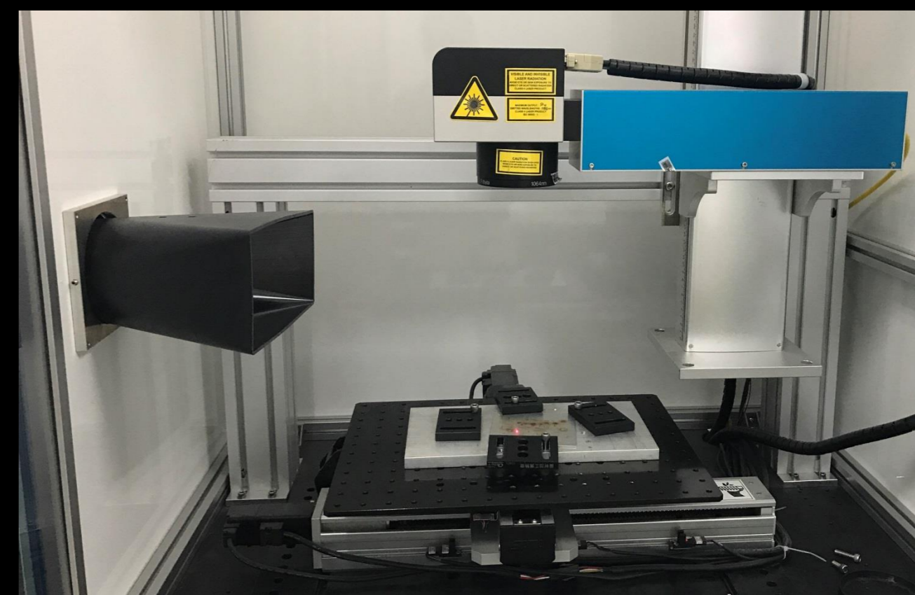
奈秒光纖雷射加工機
